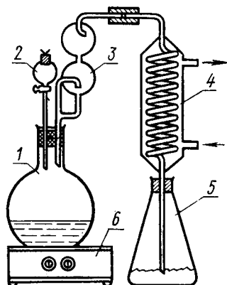
1—дистилляционная колба; 2—капельная воронка; 3—дефлегматор; 4—холодильник; 5—приемная колба; 6—электроплитка.
